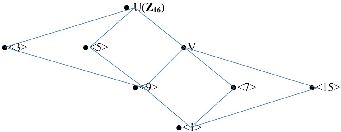
Il reticolo dei sottogruppi del gruppo U(\mathbf{Z}_{16}) degli elementi invertibili dell'anello (\mathbf{Z}_{16}, +, \cdot) .
