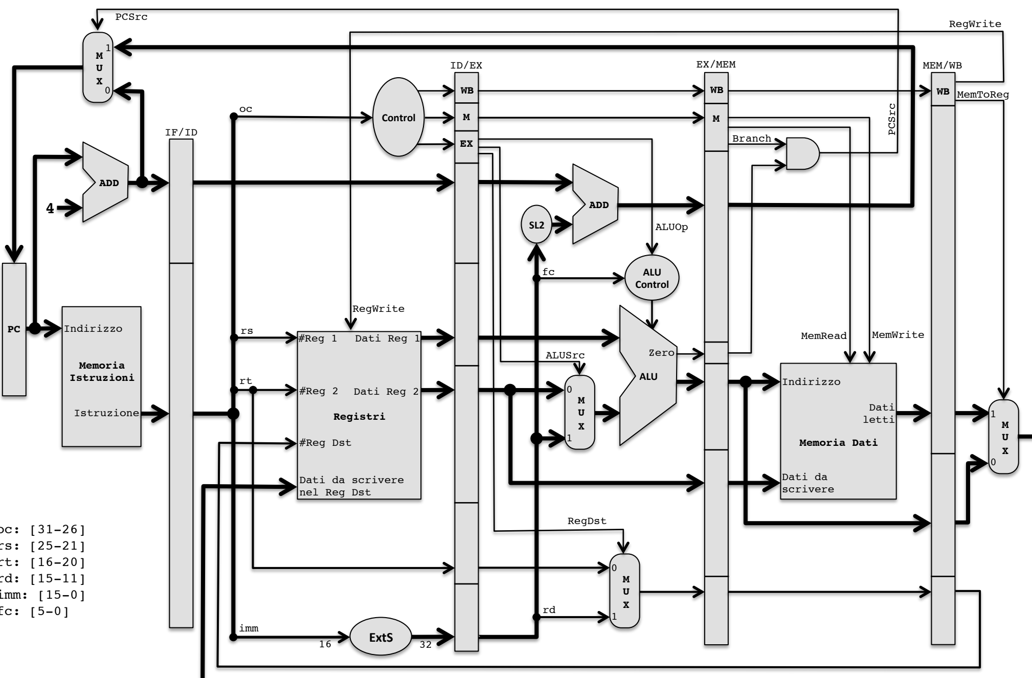
Datapath e controllo dell'implementazione in pipeline di MIPS (solamente le istruzioni di base), senza meccanismi per risolvere hazards (dati e branch).
