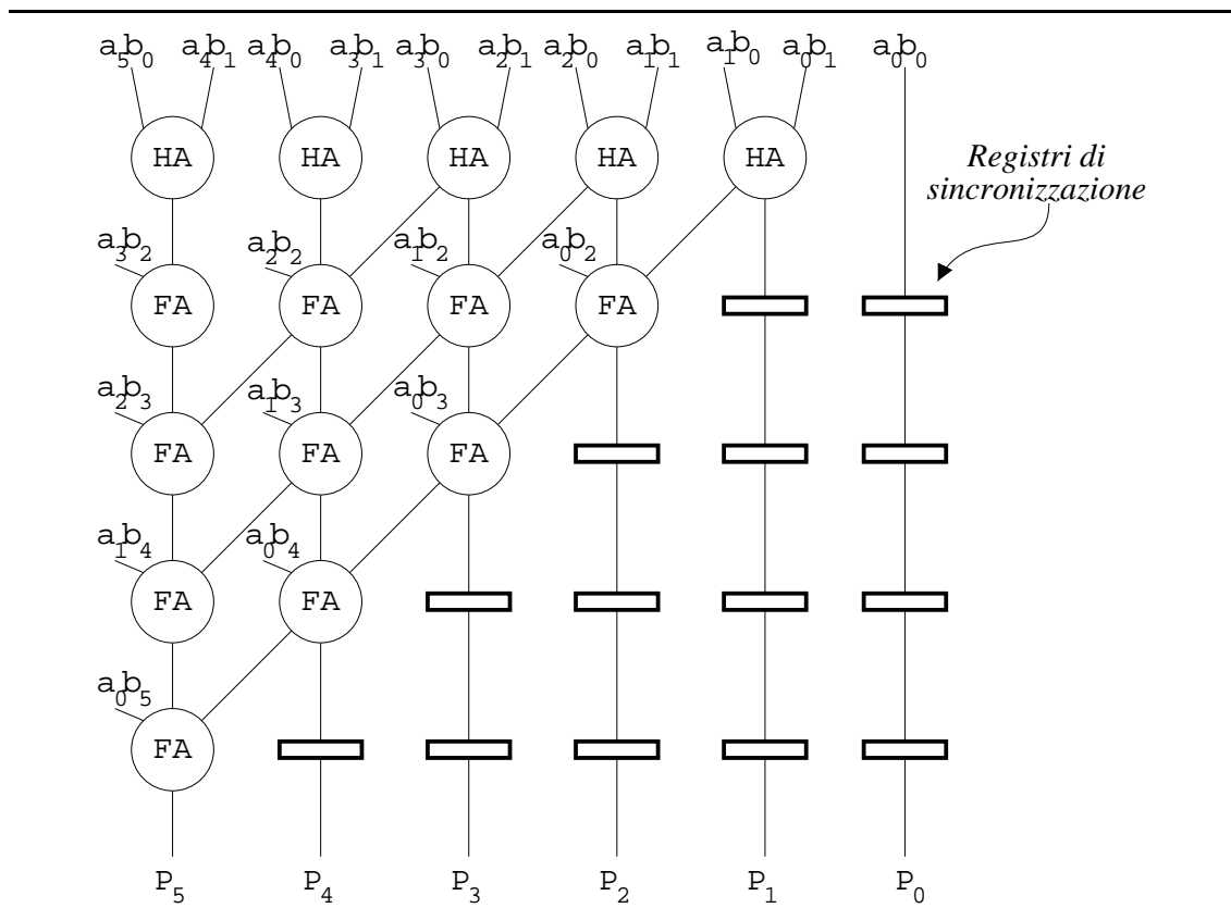
Figura 25: Moltiplicatore canalizzato per numeri in complemento a due
